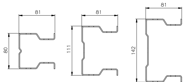
חתך עמוד בודד
