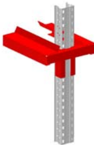
זרוע דו צדדית מורכבת על עמוד + קורת מטען
