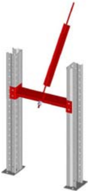
חיבור קושרת לעמוד ולמותחן
