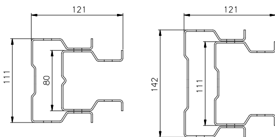
חתך עמוד כפול
